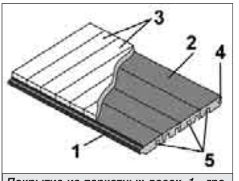
Покрытие из паркетных досок. 1 - гребень; 2 - реечный щит; 3 - лицевое покрытие из паркетной доски; 4 - паз; 5 - продольные пропили.
