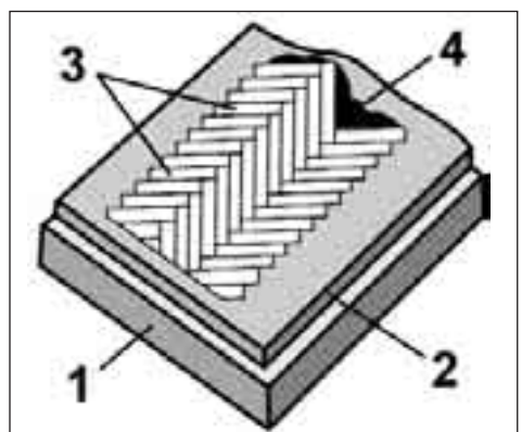
Покрытие из штучного паркета. 1 - железобетонная плита; 2 - стяжка из раствора; 3 - паркетные планки, уложенные «елкой»; 4 - битумная мастика.
