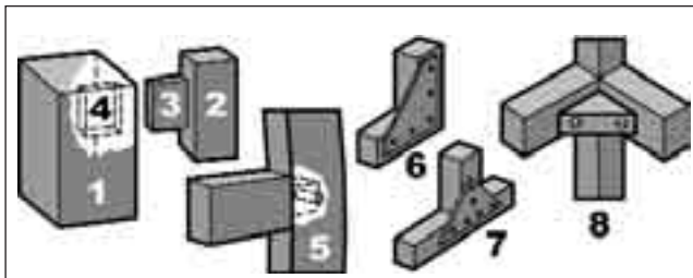
1 - ножка; 2 - царга; 3 - шип; 4 - проушина; 5 - установка деревянного гвоздя (шканта); 6, 7 - образцы накладок из фанеры; 8 - установка деревянного уголка (бонышки).
